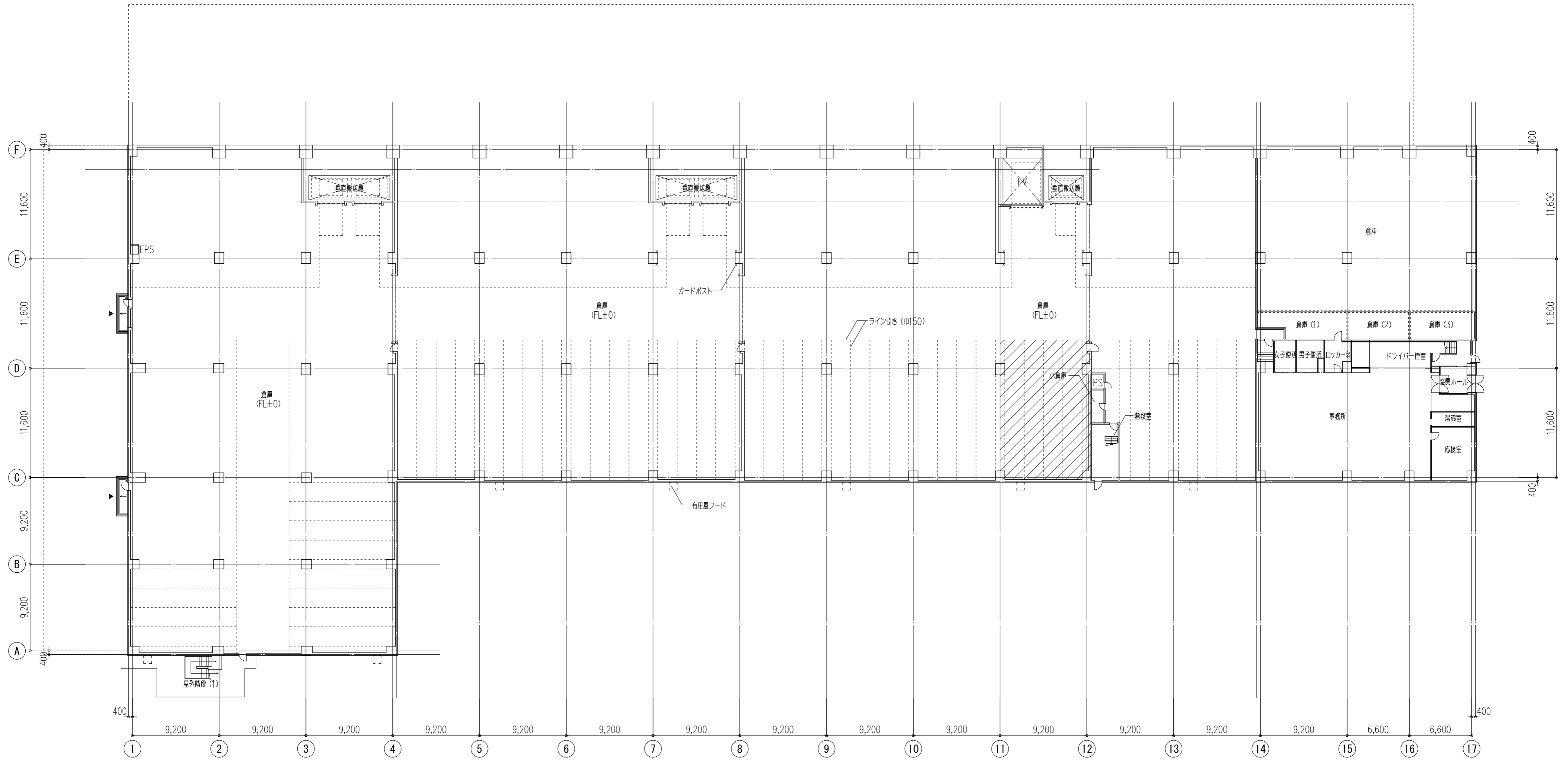
1階平面図
